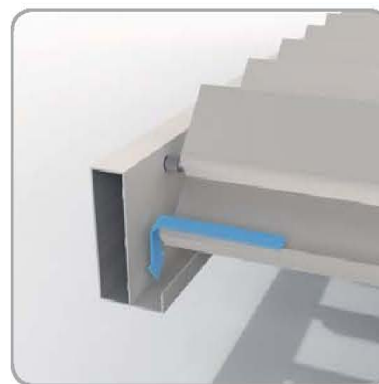
排水槽
