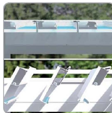
当百叶片雨后再次开启时，设计精巧的排水系统确保板积水不会产生滴漏现象
